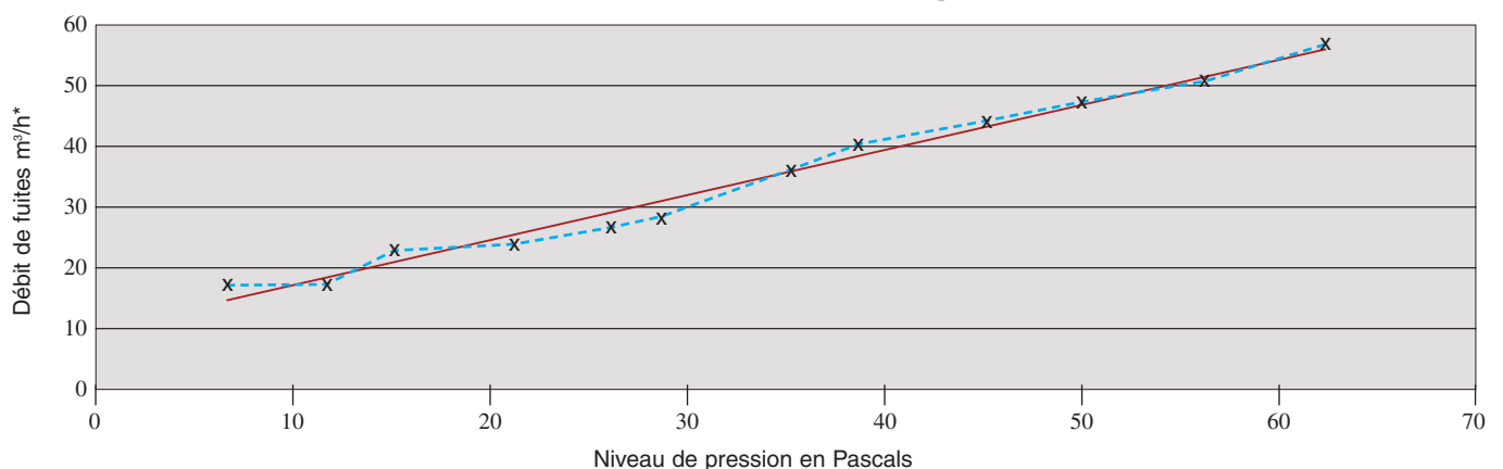
Evolution du débit de fuite en fonction du niveau de pression d'air
