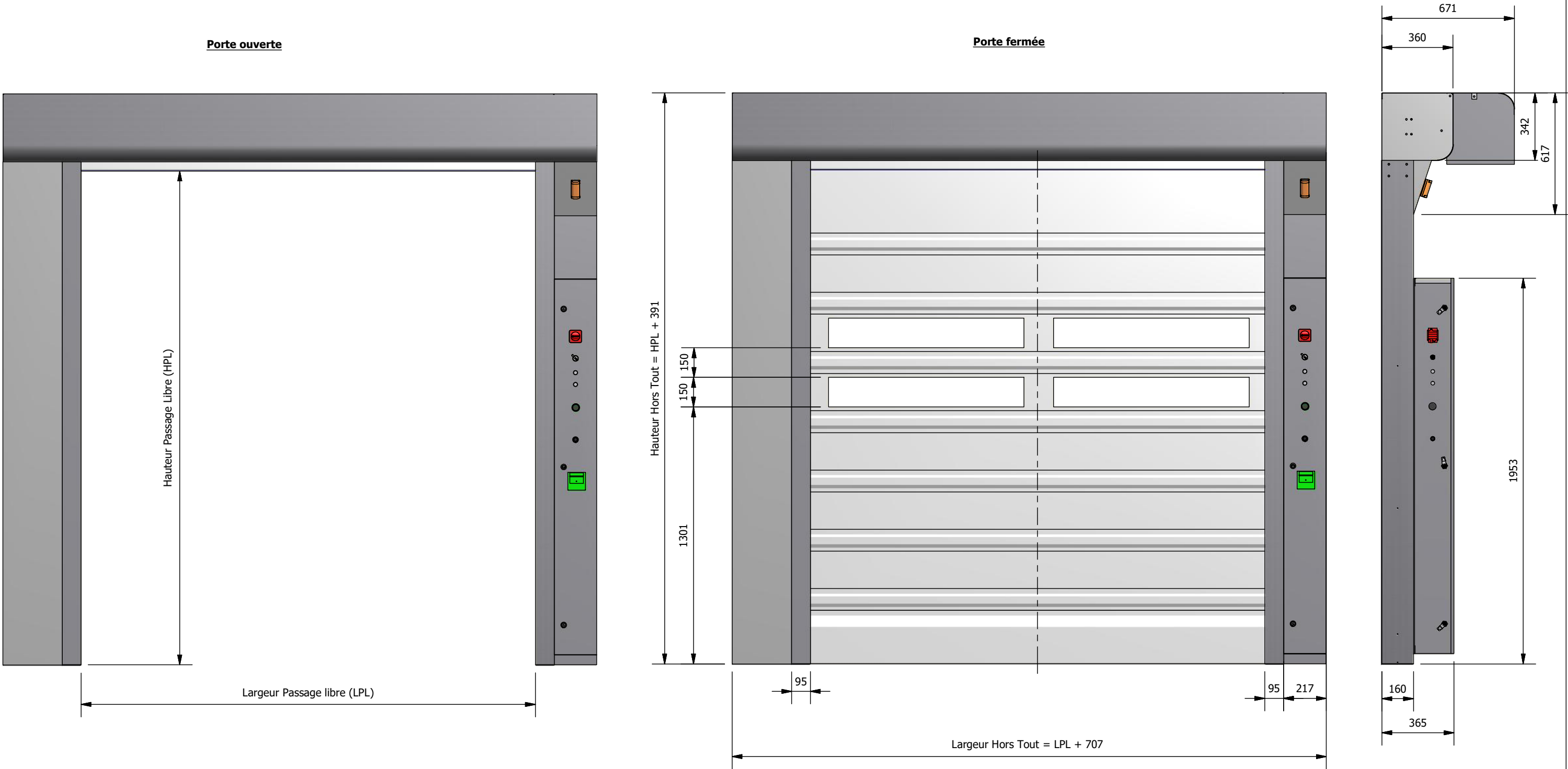
Porte symétrique avec moteur à gauche
